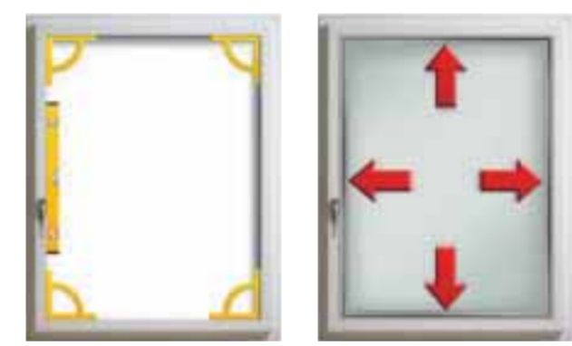
Der verschweisste Flügelrahmen wird winkelig gespannt.
